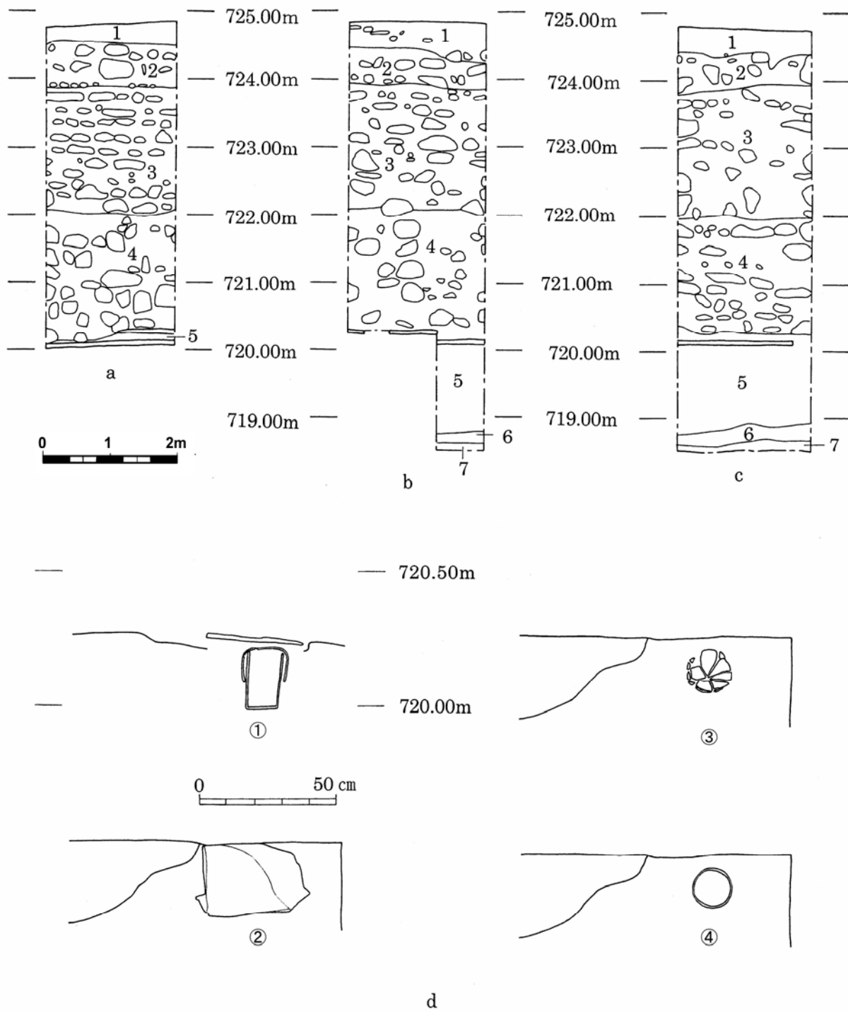
Figura 9 Cortes de Pozo 15 y Corte y Plano de la Ofrenda: Cortes: a= Oeste, b= Norte, c= Este; Ofrenda (d): ① = Corte, ② = plano de la ofrenda, ③ = vasija (tapadera), ④ = vasija cilíndrica
