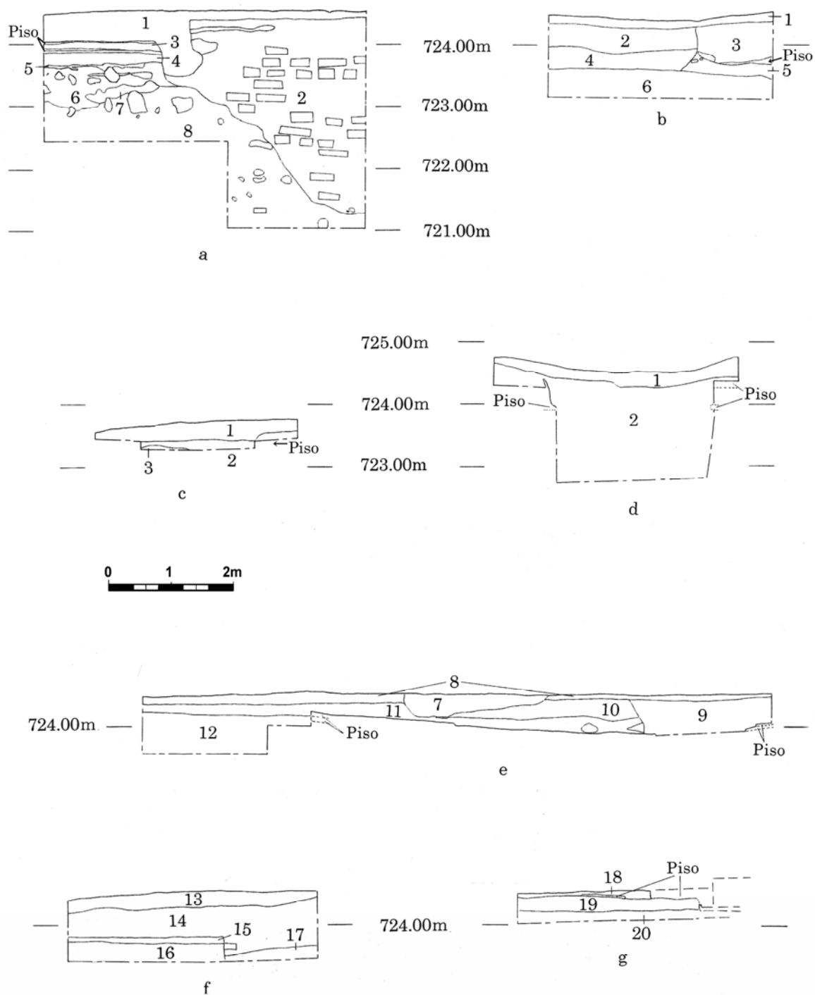
Figura 5 Cortes del Pozo 6: a= Corte Este (Pozo 6), b= Corte Oeste (Ext. Norte), c= Corte Sur (Ext. 2), d= Corte Oeste (Ext. 3), e= Corte Oeste (Ext. Oeste 4-7, 9), f=Corte Oeste (Ext. Oeste 8), g= Corte Sur (Ext. Oeste 1)
