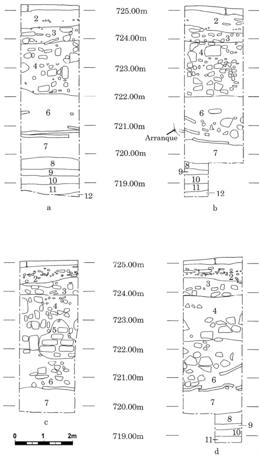
Figura 8 Cortes de Pozo 17: a= Norte, b=Este, c= Sur, d= Oeste
