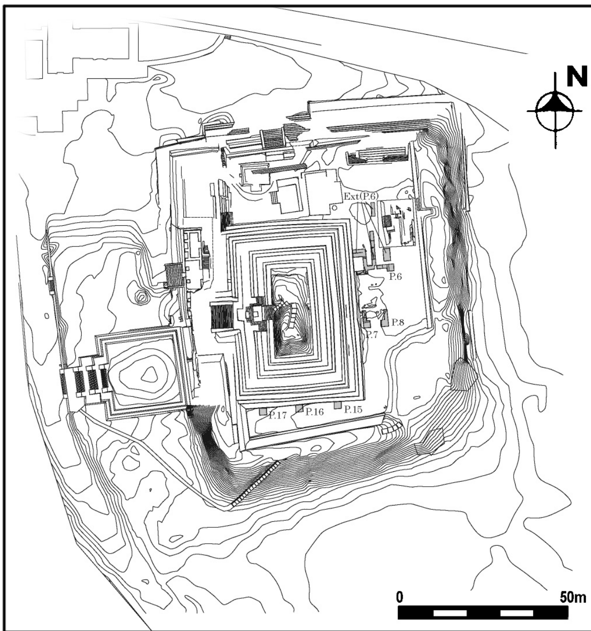
Figura 4 Pozos 6-8, 15-17 en el Parque Arqueológico de Tazumal
