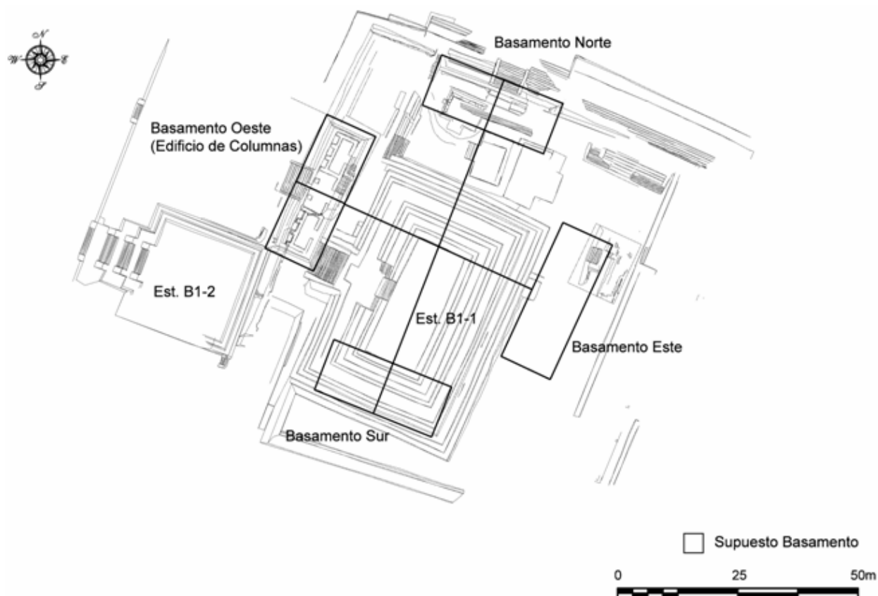
Figura 3 Supuestos Basamentos en la Estructura B1-1
