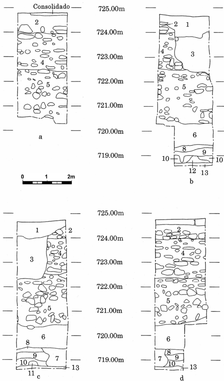
Figura 7 Cortes del Pozo 16: a= Norte, b=Este, c= Sur, d= Oeste
