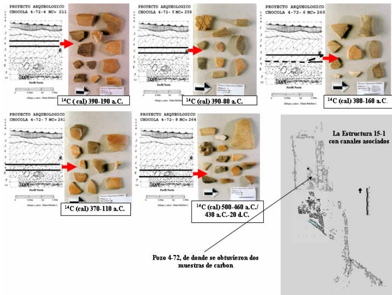
Figura 8 Fechas de radiocarbono de estratos superiores al canal del sistema hidráulico
