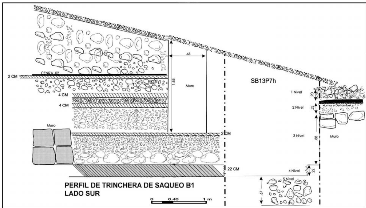
Figura 6 Perfil sur de trinchera de saqueo B1
