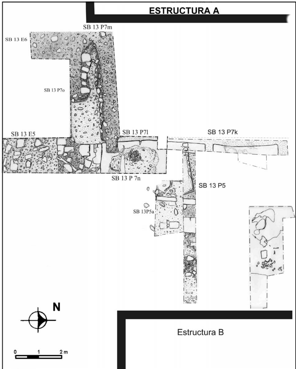
Figura 17 Planta de las Suboperaciones de Patio 1
