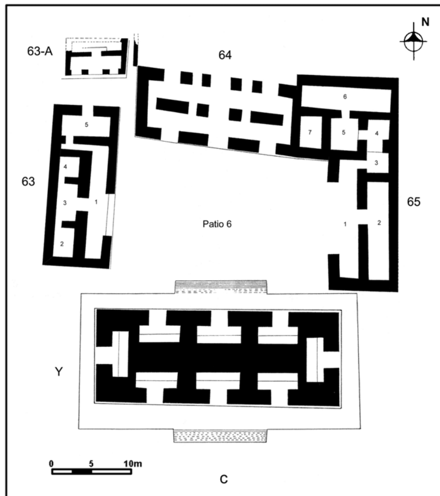
Figura 8 Planta del Edificio F durante el Clásico Tardío (estadio F-2, [a]) y durante el Clásico Terminal (estadio F-2b [b]). Planta del Patio 6 con ubicación de los Edificios Y, 63, 63-A, 64 y 65 (c)
