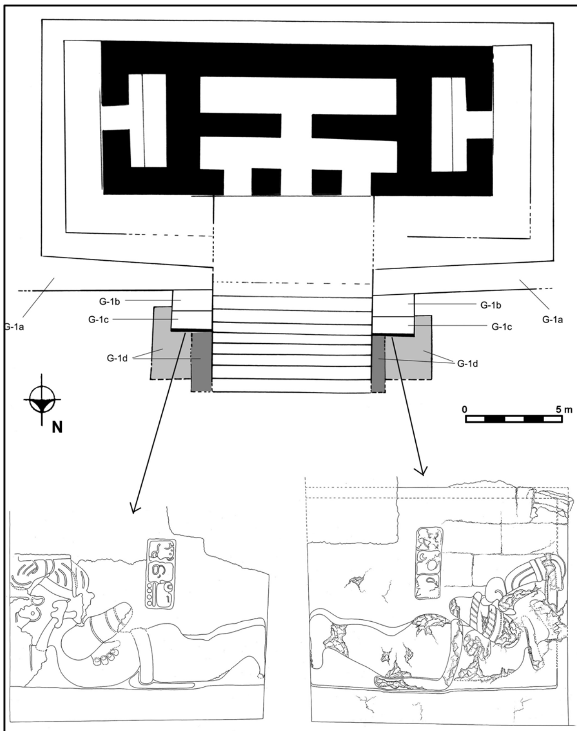
Figura 6 Planta del primer nivel del Edificio G marcando estadios constructivos y representaciones de cautivos del estadio G-1c
