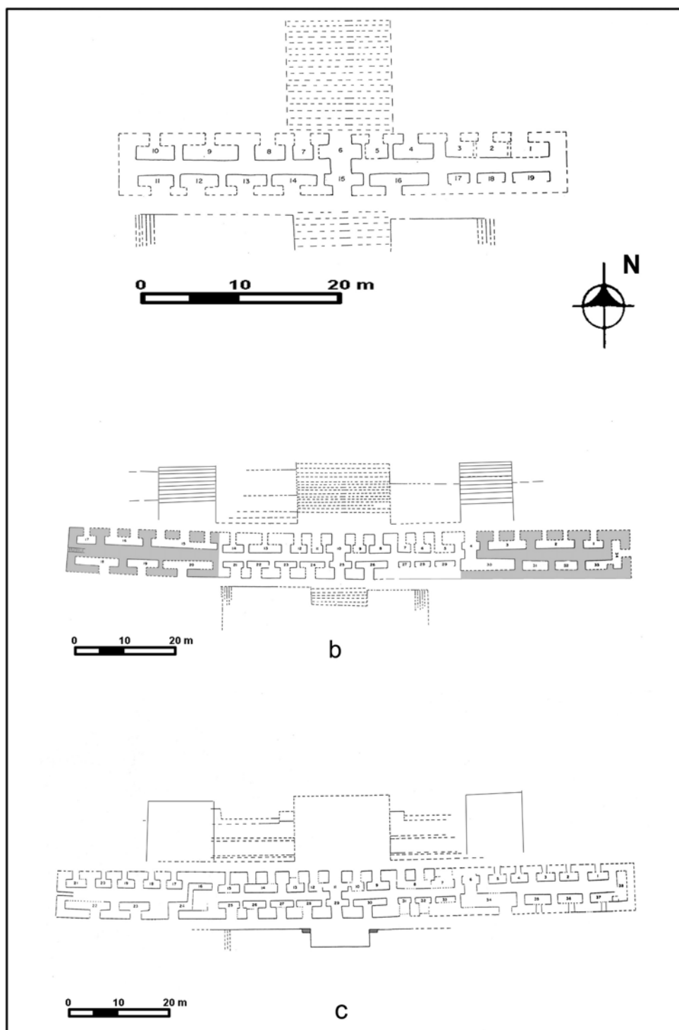
Figura 4 Edificio D, planta de estadios constructivos del Clásico Tardío (a) y Clásico Terminal (b y c)
