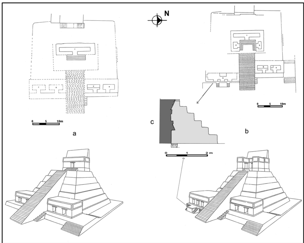
Figura 5 Edificio E, planta e idealización del último estadio constructivo del Clásico Tardío (a) y primer estadio del Clásico Terminal (b) con corte de perfil talud-tablero-cornisa volada (c)
