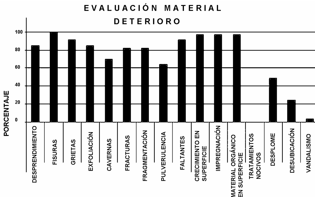
Figura 8 Análisis de los deterioros de los monumentos de Yaxha
