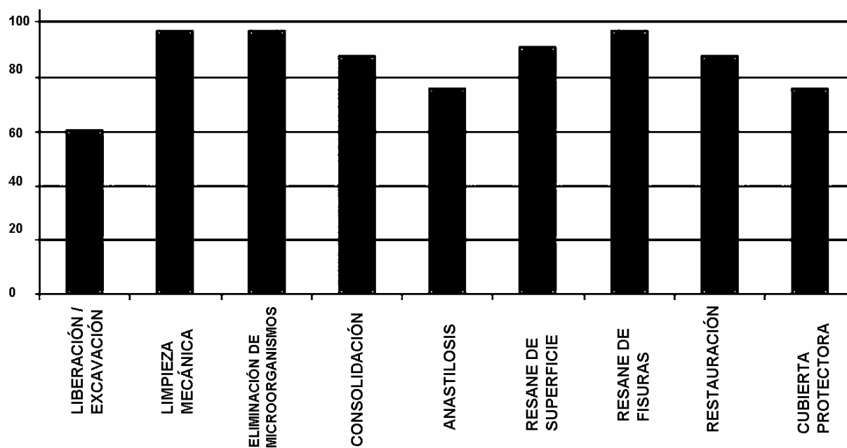
Figura 10 Análisis cuantitativo de la intervención propuesta
