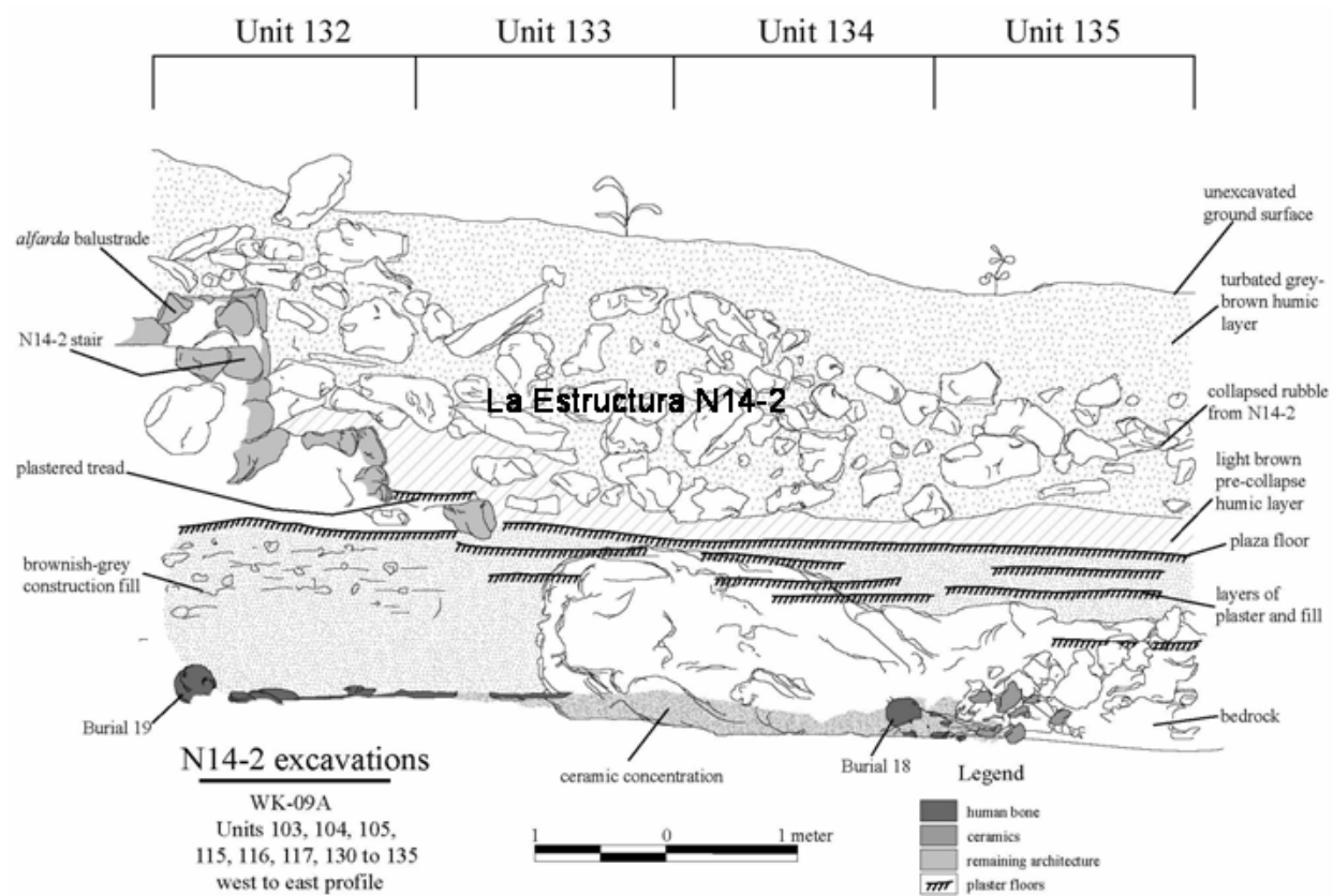
Figura 1 Corte de la Estructura N14-2
