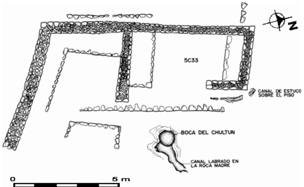
Figura 4 Plano de la Estructura 5C33
