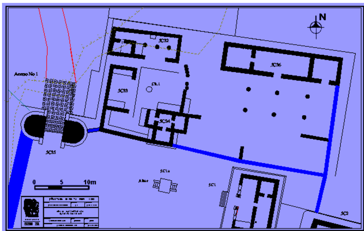
Figura 9 Estructuras del Grupo de La Serie Inicial
