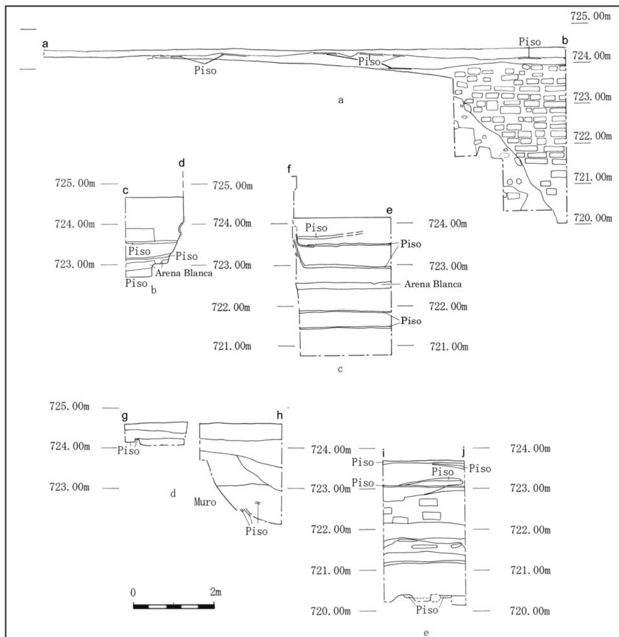
Figura 7 Cortes en la Parte Norte de la Estructura B1-1, Tazumal. a: Perfil Norte del Trincheras 23 (a-b), b: Perfil Este del Pozo 25 Ext. Sur (c-d), c: Perfil Norte del Pozo 19 (e-f), d: Perfil Norte del Pozo 21 (g-h), e: Perfil Este del Pozo 25 (i-j).
