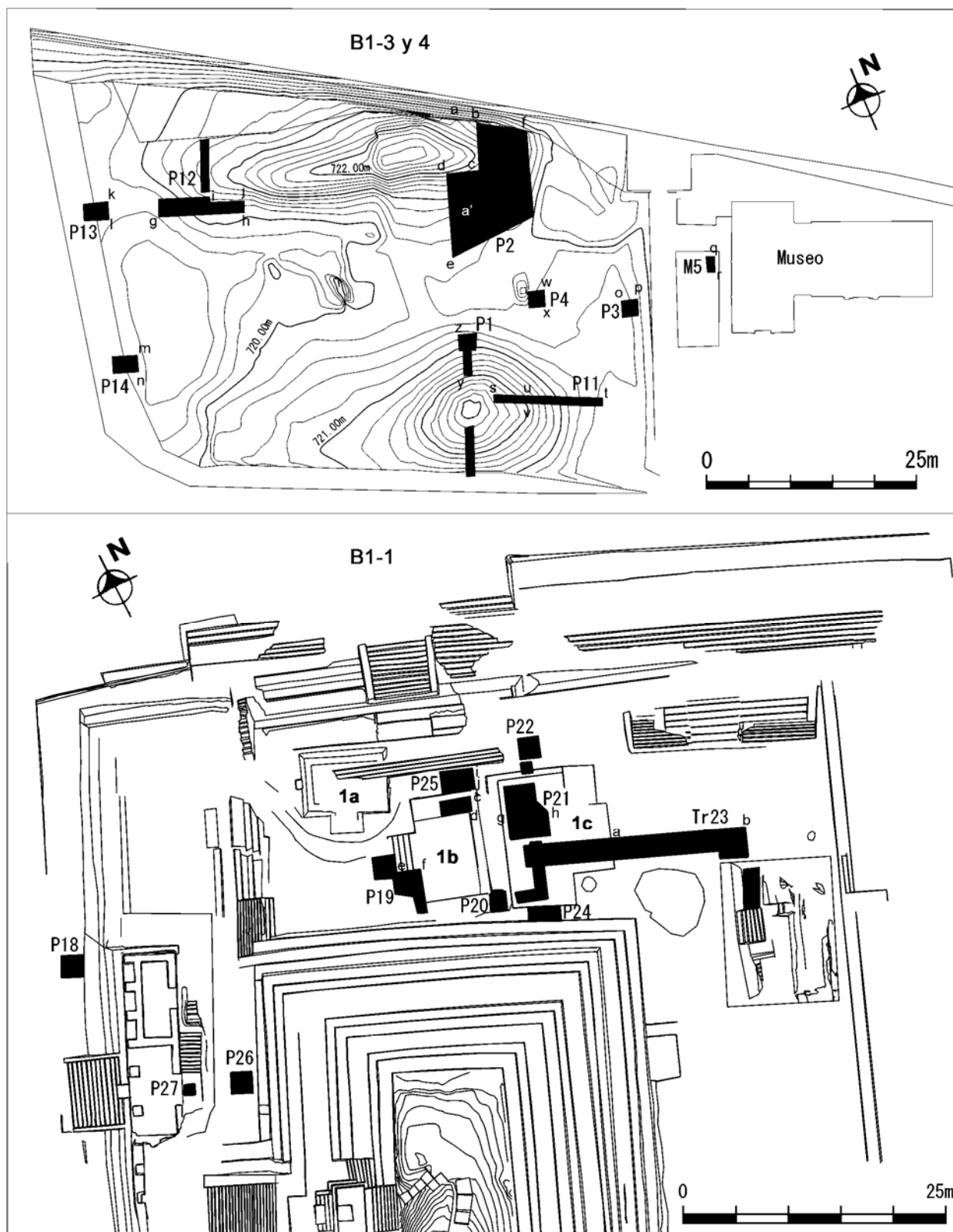
Figura 2 Pozos y la Trinchera en la Estructura B1-1, 3 y 4, Tazumal
