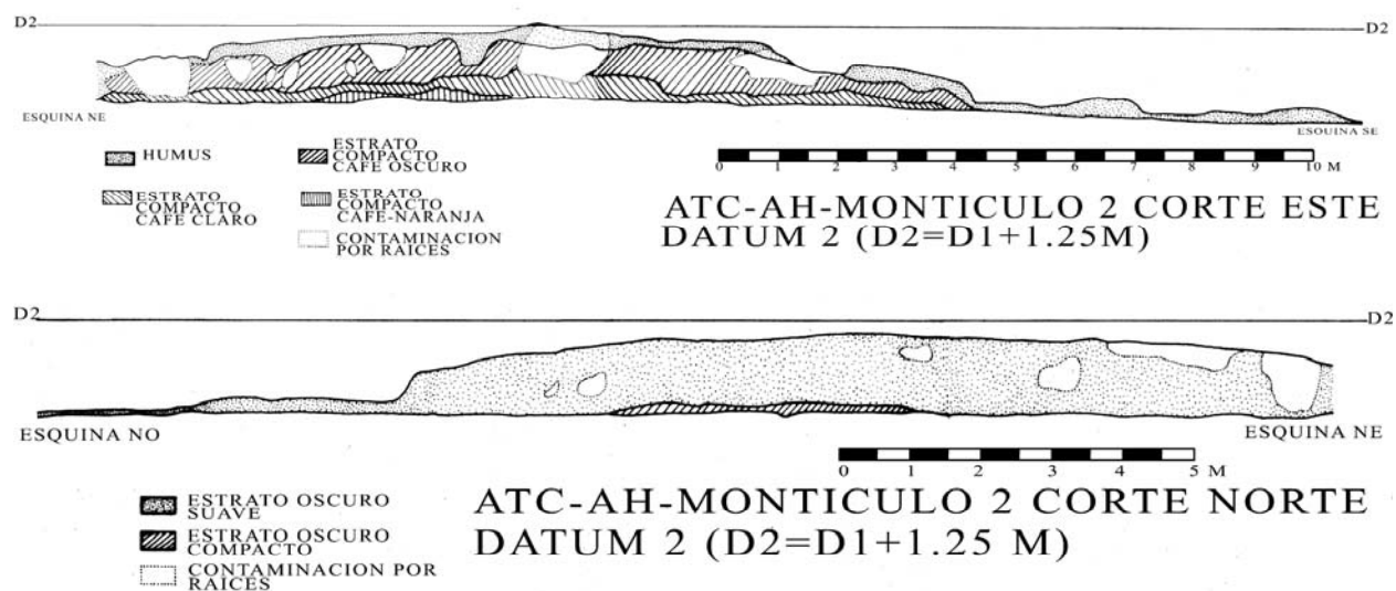
Figura 5 Ilustración de cortes Norte y Este Montículo 2
