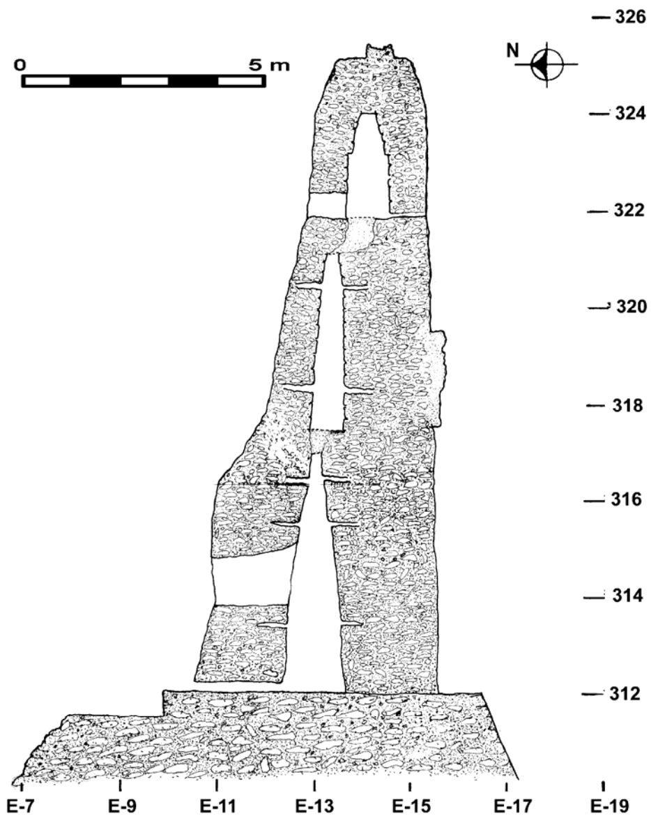
Figura 9 Sección este-oeste, cámaras 1 de tres niveles de crestería, Templo IV, Tikal
