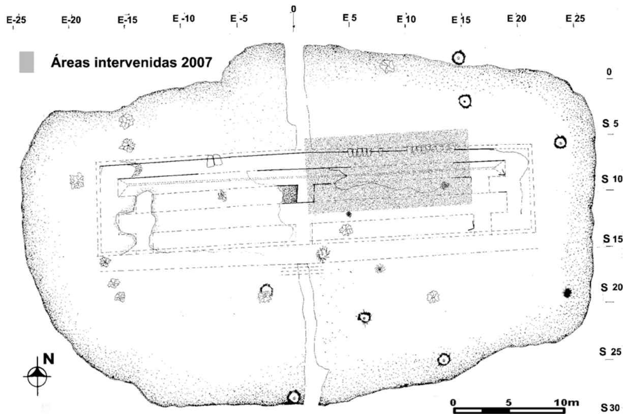
Figura 6 Planta Estructura 5D-15 con intervenciones 2007
