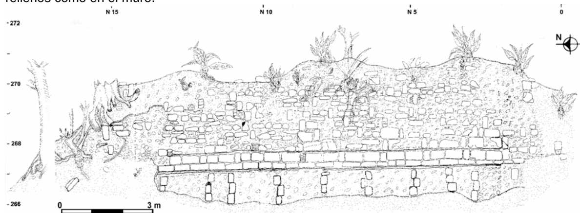
Figura 7 Elevación muro exterior Oeste, Estructura 5C-47, "La Herradura", Mundo Perdido
