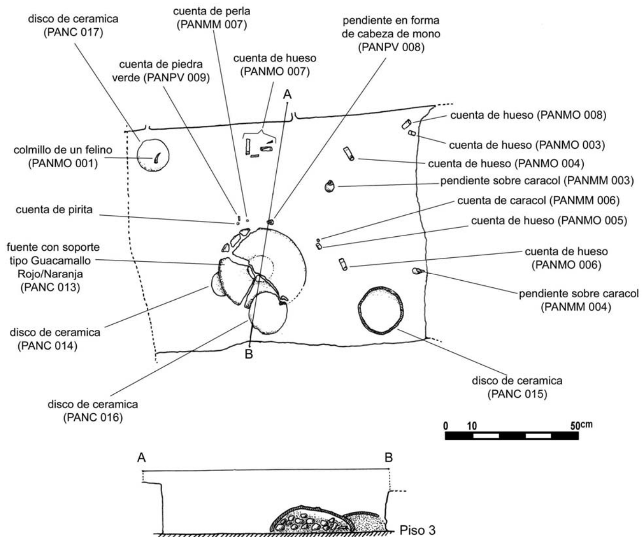
Figura 2 Planta y corte de la Ofrenda 8 de Nakum, Edificio 99 (dibujo por Aleksander Danecki)
