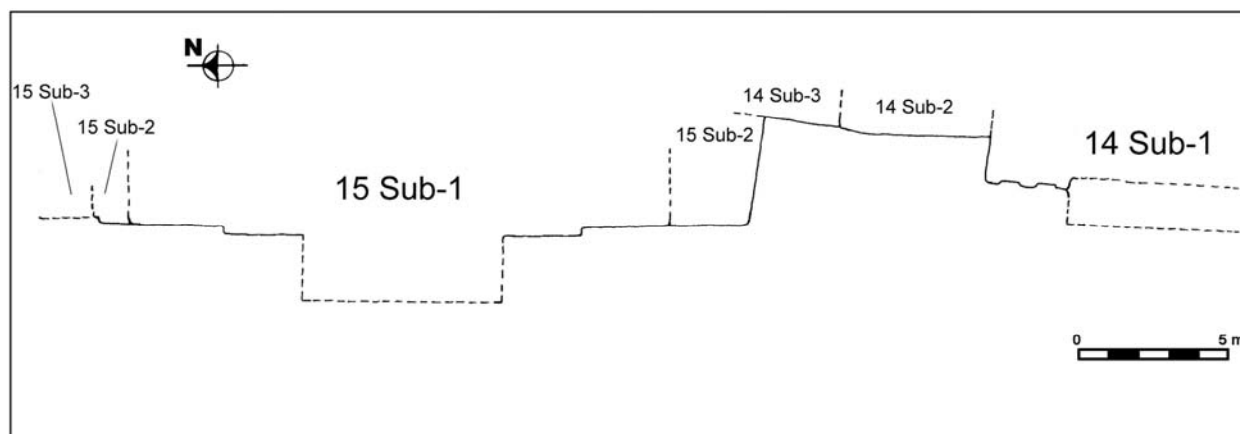
Figura 13 Planta de las fachadas de los Edificios 14 Sub 1 a 3 y 15 Sub 1 a 3. Protoclásico y Clásico Temprano (dibujo por Wiesław Koszkul)
