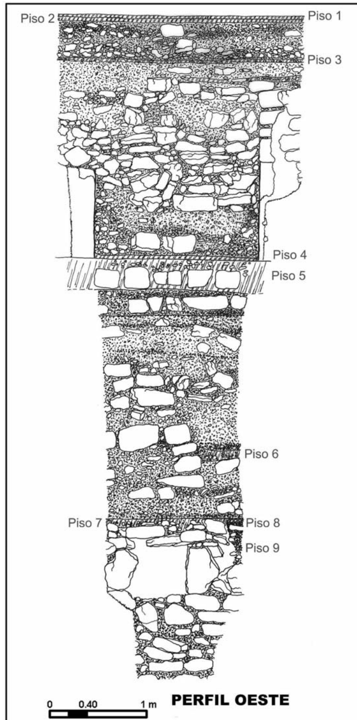
Figura 8 Perfil oeste en la Suboperación 3A, Edificio 15, Nakum. Dibujo por Wiesław Koszkuł
