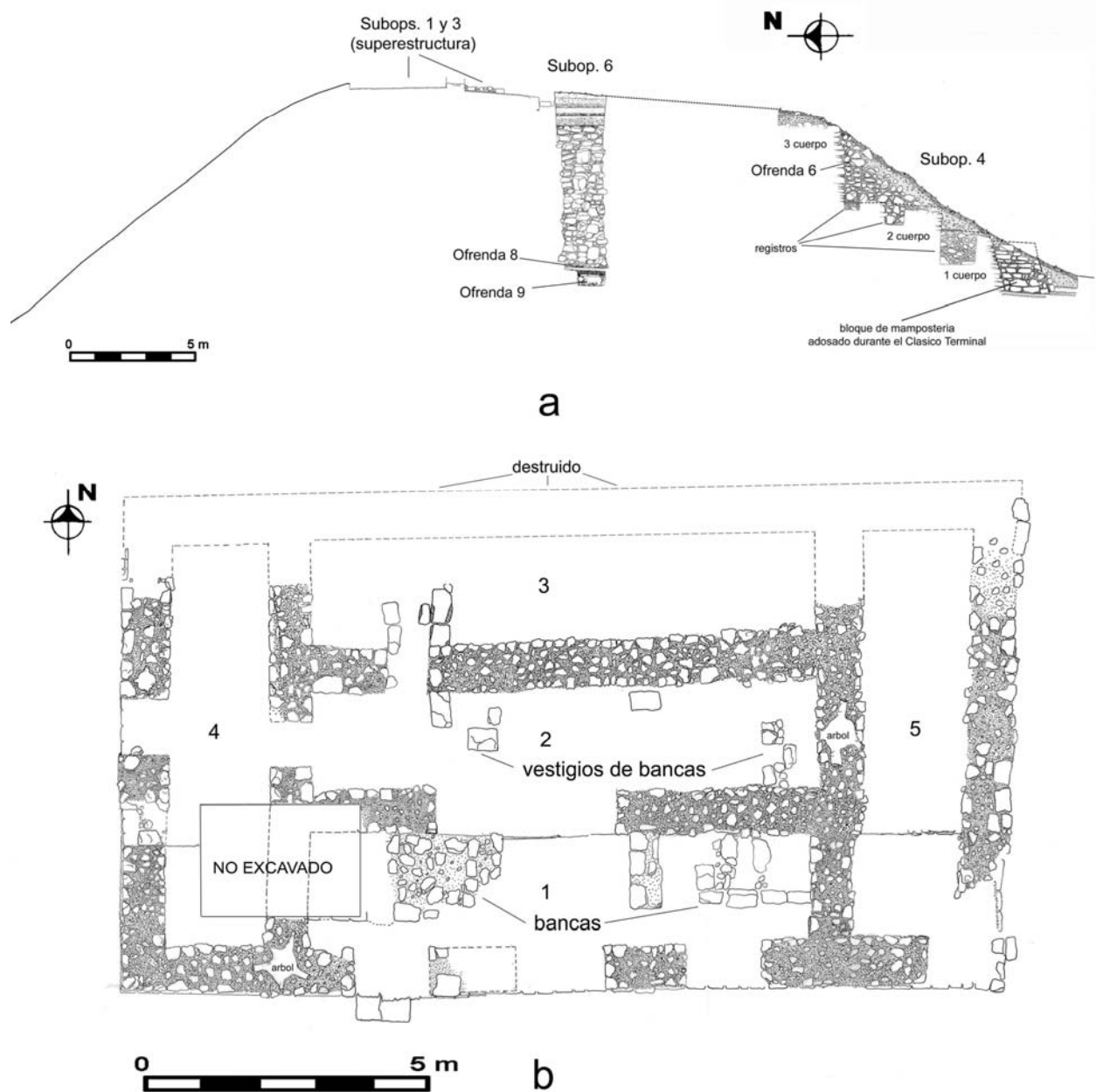
Figura 1 Edificio 99 de Nakum, a) corte norte-sur del edificio con ubicación de las excavaciones del año 2007, b) planta de la superestructura descubierta en la cumbre de la plataforma del Edificio 99 (Dibujos por Aleksander Danecki y Pawel Kurzawa)
