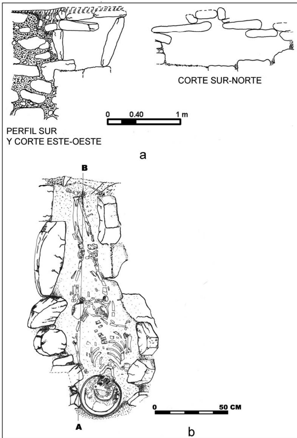
Figura 9 Entierro 2, Edificio 15, Nakum (dibujo por Wiesław Koszkuł y Bogumił Pilarski)
