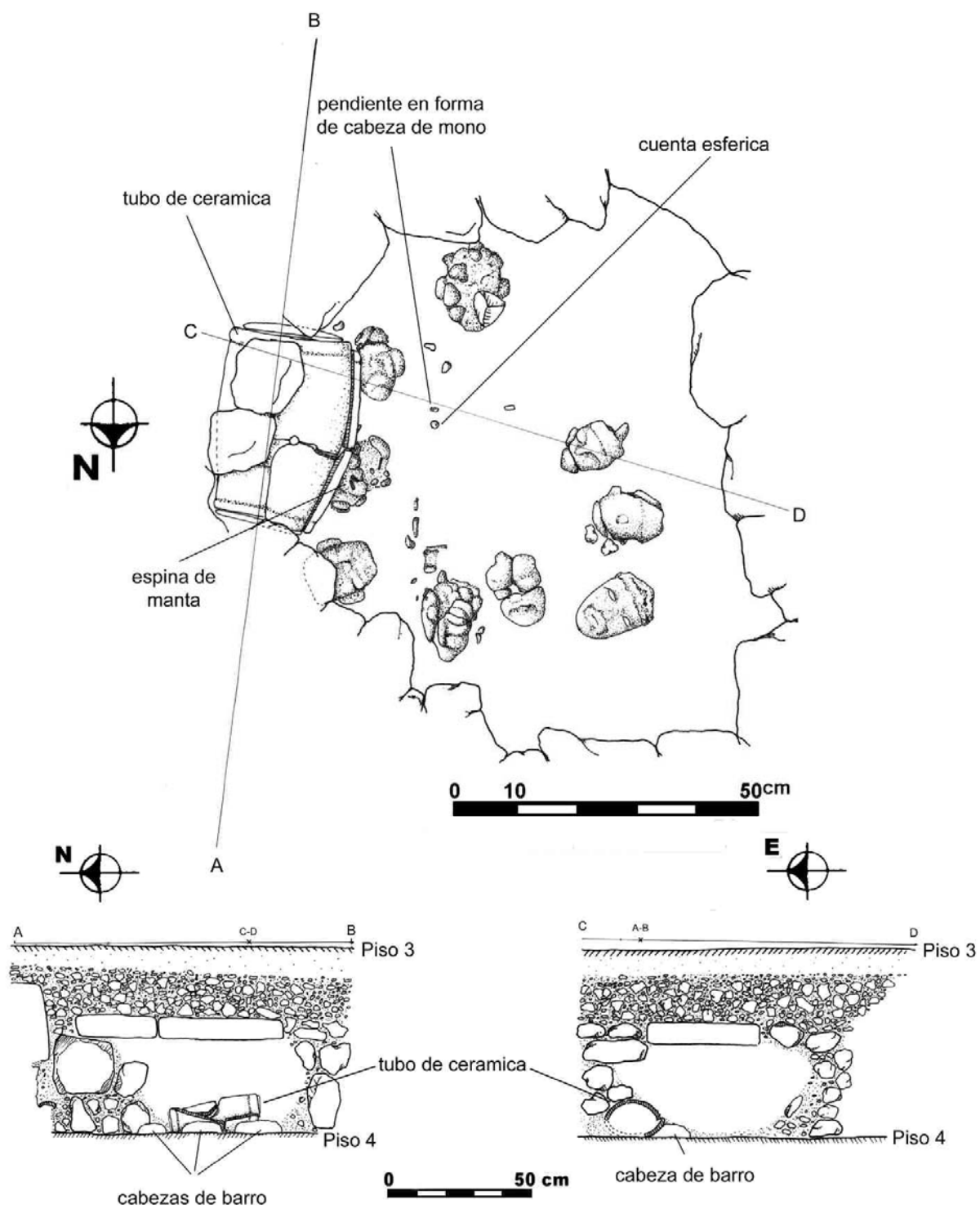
Figura 3 Planta y cortes de la Ofrenda 9 de Nakum, Edificio 99 (Dibujo por Katarzyna Radnicka y Aleksander Danecki)
