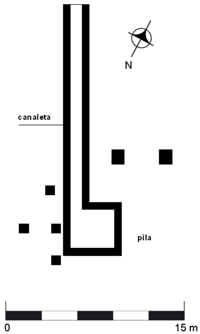
Figura 4 Plano de planta de los vestigios arqueológicos del Ingenio San Rafael, Cantón Santa Rita, Metapan. Agosto 2008. PAHES-UTEC (Dibujo Erquicia, Menjívar, Barraza, Herrera y Campos. Digital A.de Erquicia).
