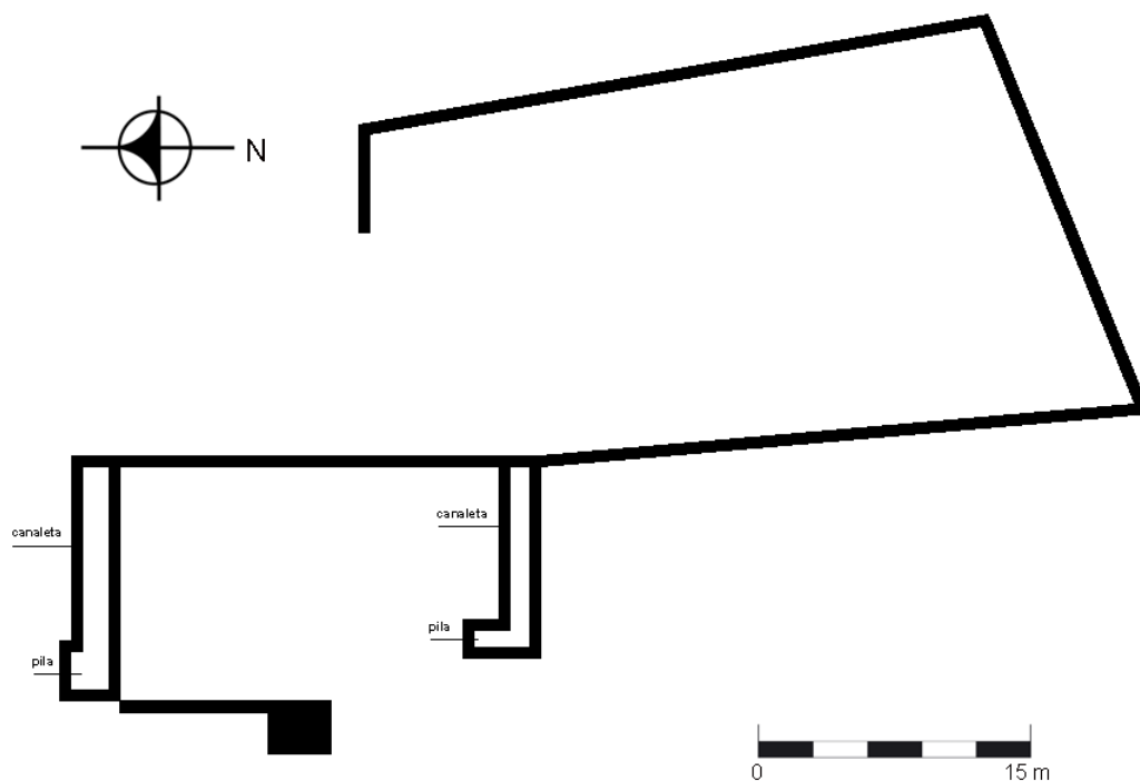
Figura 3 Plano de planta de los vestigios arqueológicos del Ingenio El Carmen, Cantón El Panal, Caserío El Carmen, Metapan. Agosto 2008. PAHES-UTEC (Dibujo Erquicia, Barraza, Herrera y Campos. Digital A.de Erquicia).
