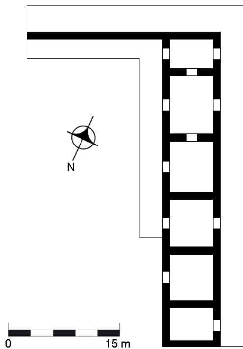
Figura 5 Plano de planta de la Antigua Hacienda Gualcho, Usulután. Agosto 2008. PAHES-UTEC. (Dibujo Erquicia, Menjívar, Herrera y Campos. Digital A.de Erquicia).
