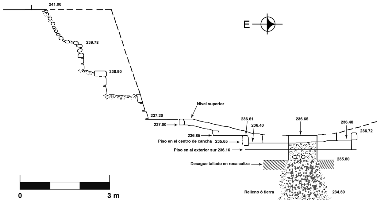
Figura 7 Corte E – O drenaje al sur de cancha Juego de Pelota 1.
