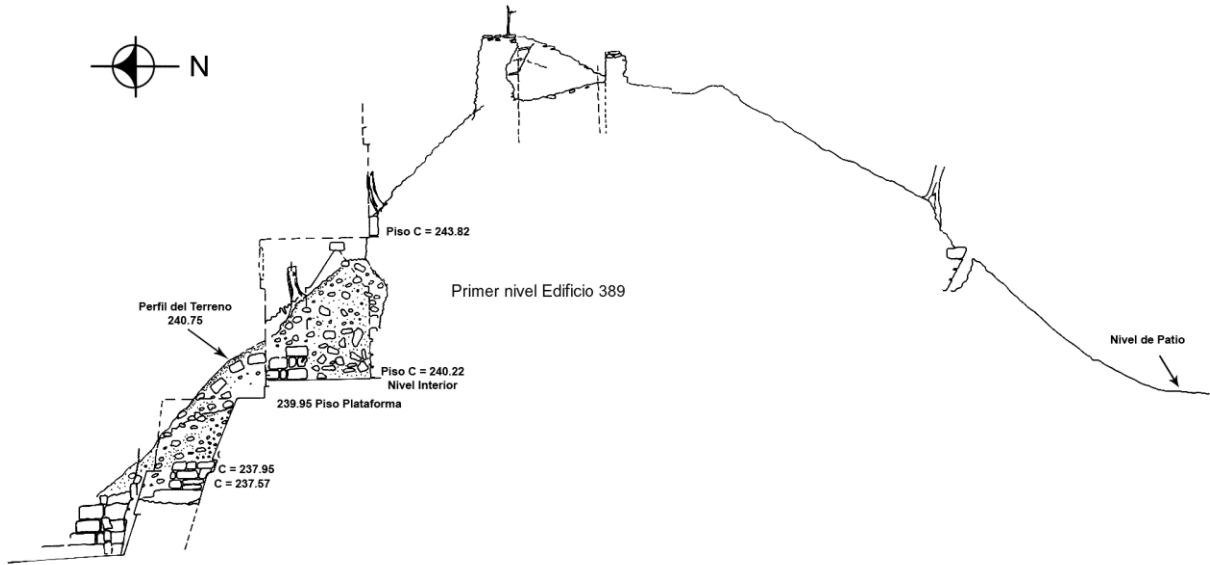
Figura 5 Corte N – S basamento lado norte Acrópolis Sur y Edificio 389.
