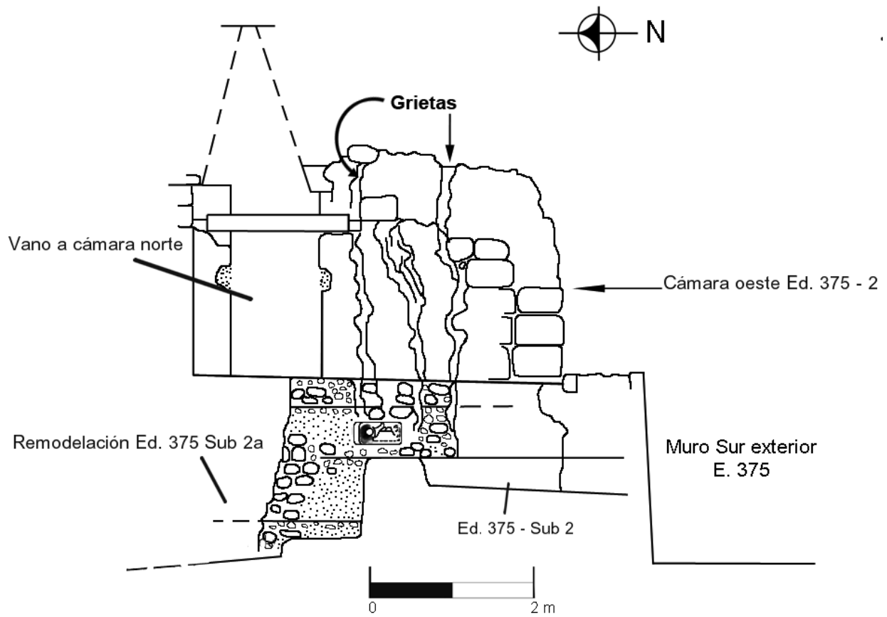
Figura 14 Corte N – S Edificio 375 mostrando Ed 375 Sub 2 y Sub 2a.
