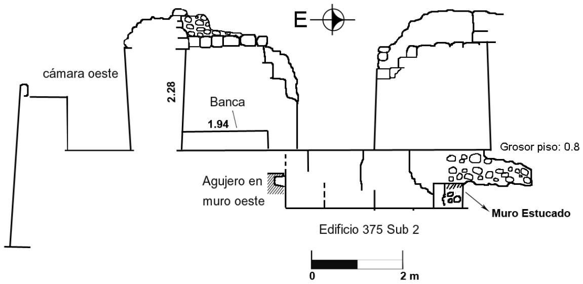
Figura 13 Corte E – O Ed. 375 mostrando Ed. 375 Sub 2.
