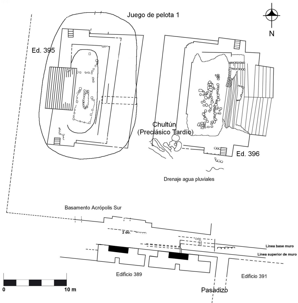
Figura 6 Planta Juego de Pelota 1, Edificio 389 y lado norte basamento Acrópolis Sur.
