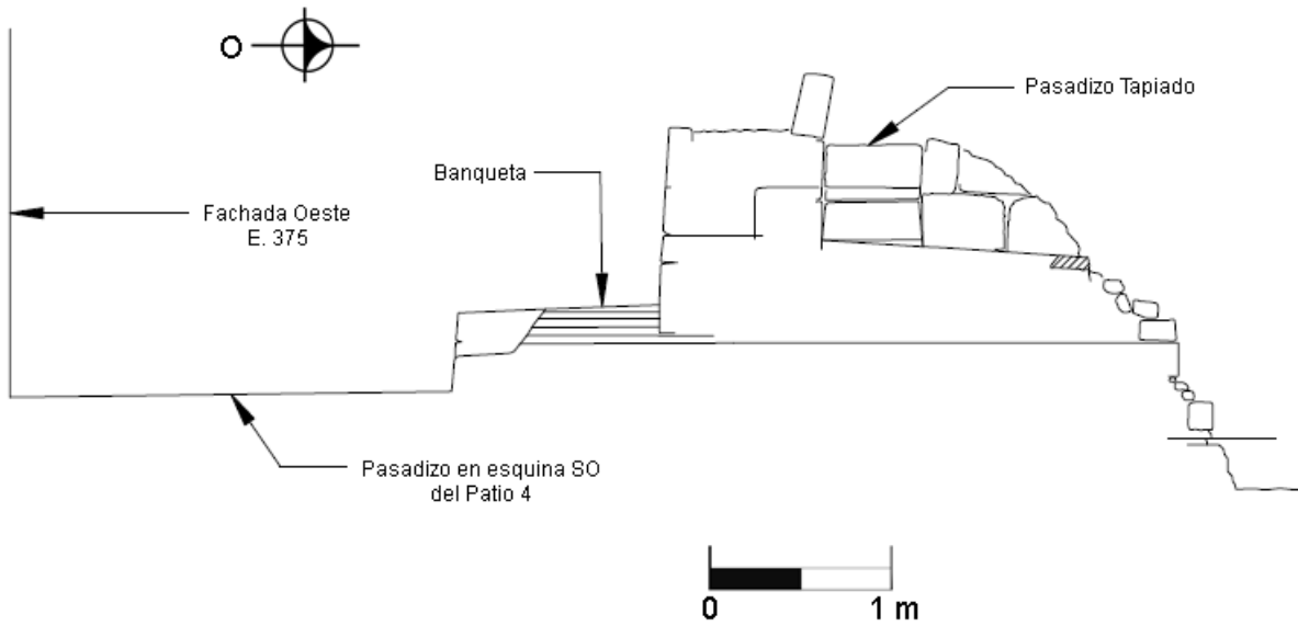
Figura 10 Corte E - O Edificio 372, límite oeste Patio 4 Acrópolis Sur.
