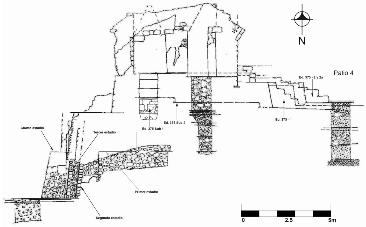
Figura 8 Corte N – S lado sur basamento Acrópolis Sur y Edificio 375.
