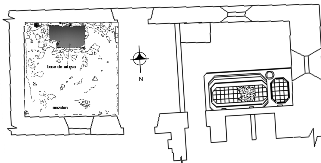
Figura 5 Conjunto de la artesa en el actual ingreso al monumento (Dibujo C. Martínez, calco L. Gómez).
