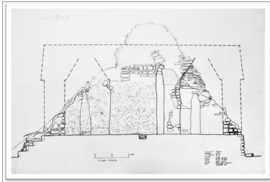
Figura 4 Perfil de las cámaras centrales que conforman el axis este-oeste del Edificio B-18, del sitio Naranjo (Dibujo V. Orellana).
