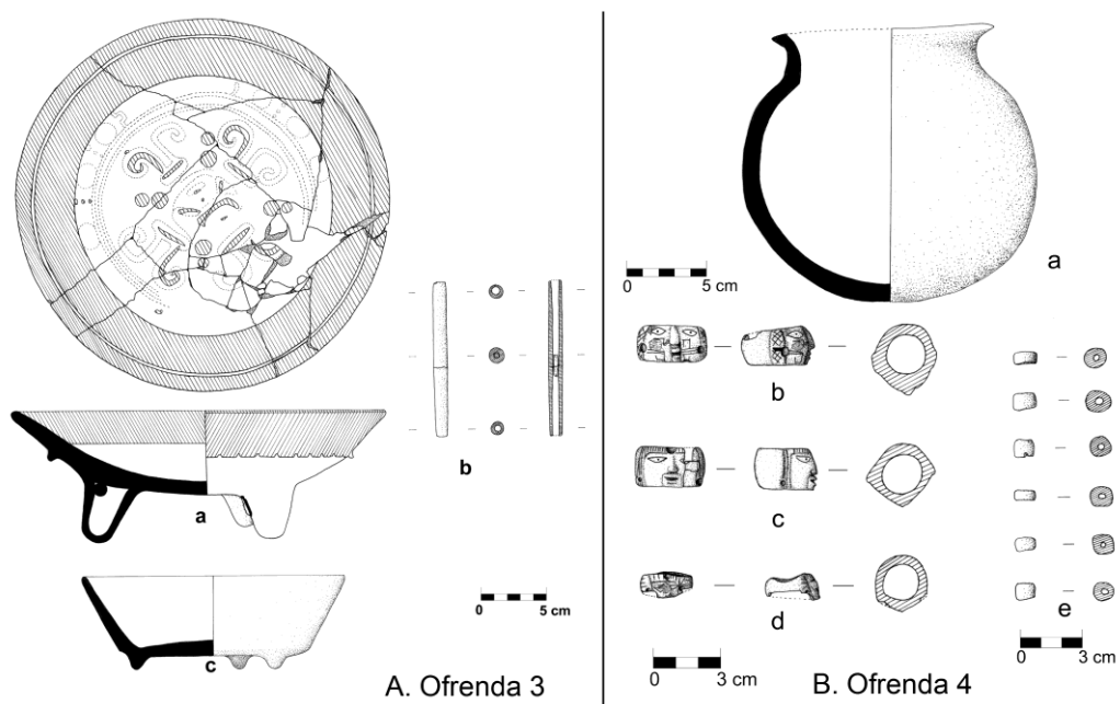
Figura 3 Ofrendas 3 y 4 descubiertos en el Edificio 15 de Nakum (Dibujo por K. Radnicka) A. Ofrenda 3 se fecha para el Clásico Tardío; B. Ofrenda 4 para el Clásico Terminal.
