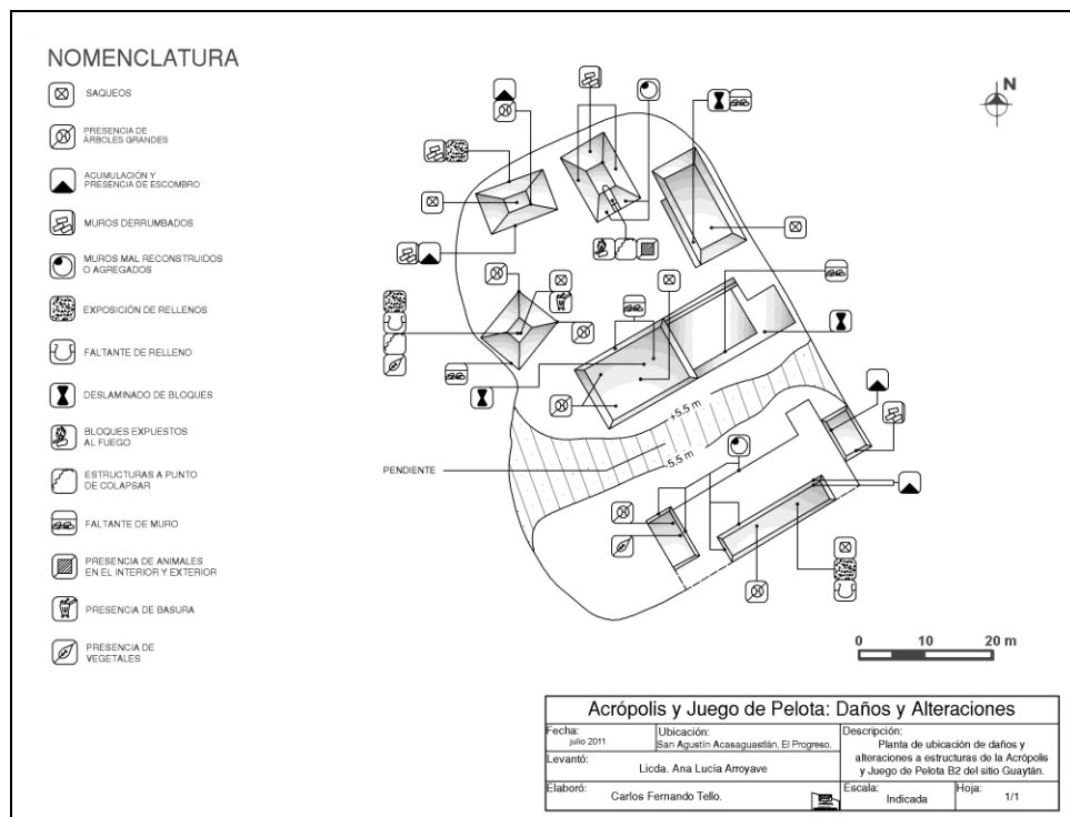
Figura 4: Planta de daños y alteraciones.
