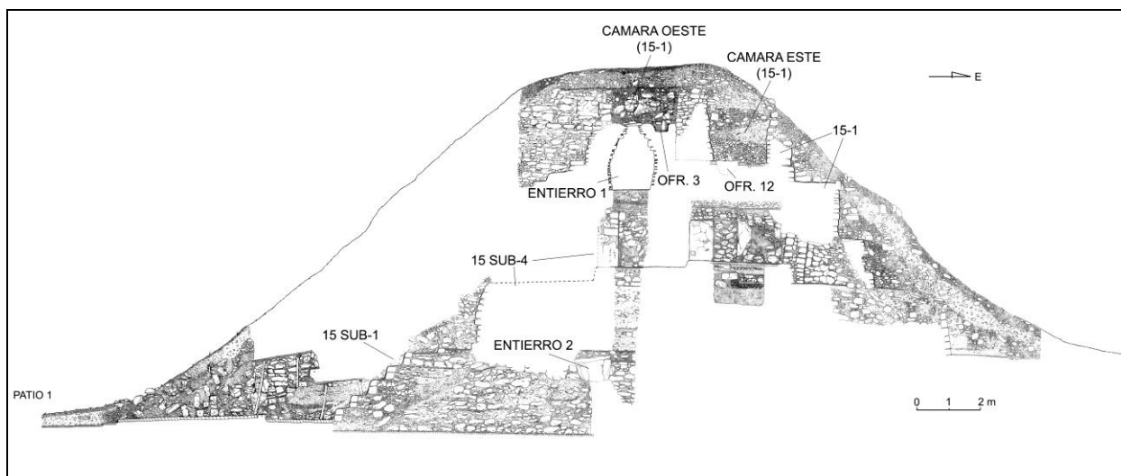
Figura 4. Corte E-O del Edificio 15 de Nakum; visibles son los mayores estadios constructivos, entierros y ofrendas. Dibujo por Wiesław Koszkuł, Bogumił Pilarski y Katarzyna Radnicka.
