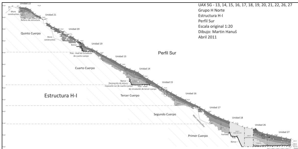
Figura 3. Perfil de la trinchera sobre la fachada oeste de la Estructura H-I (dibujo por Martin Hanus).
