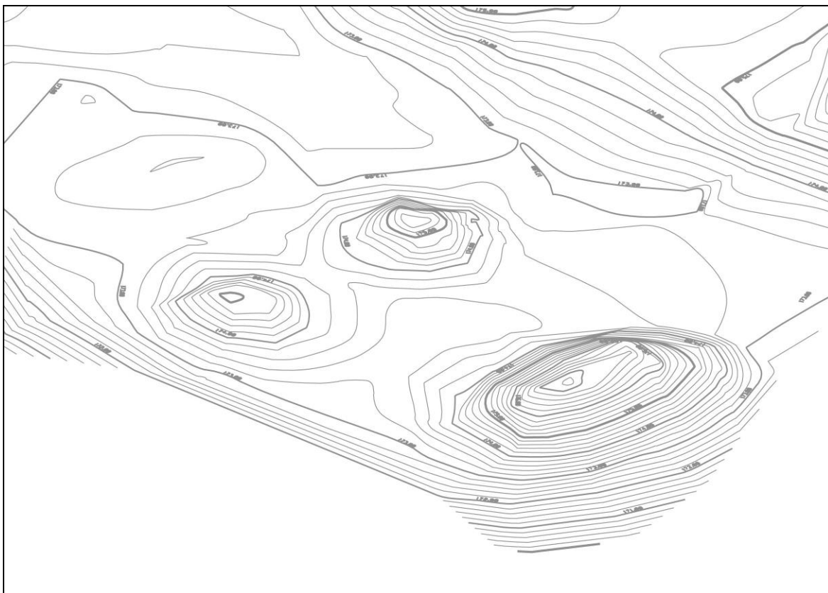
Figura 4. Levantamiento topográfico del Juego de Pelota preclásico, Grupo H Sur.
