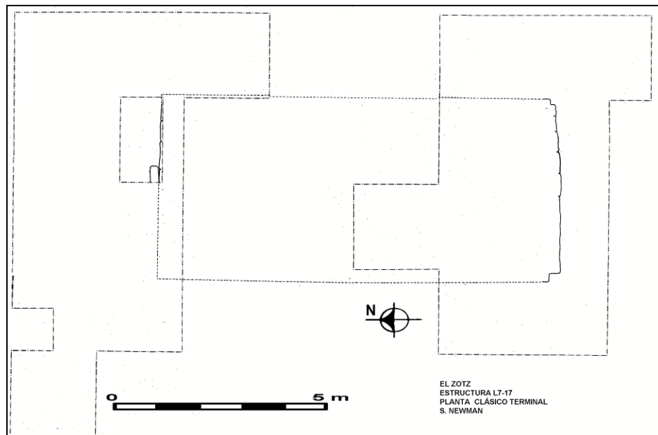
Figura 7. Planta de la estructura del Clásico Tardío debajo de la Estructura L7-17 (Dibujo: S. Newman).
