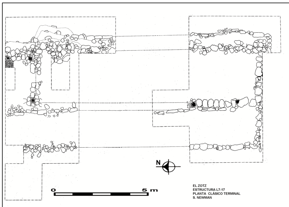
Figura 8. Planta de la forma de la Estructura L7-17 durante el periodo Clásico Terminal (Dibujo: S. Newman).
