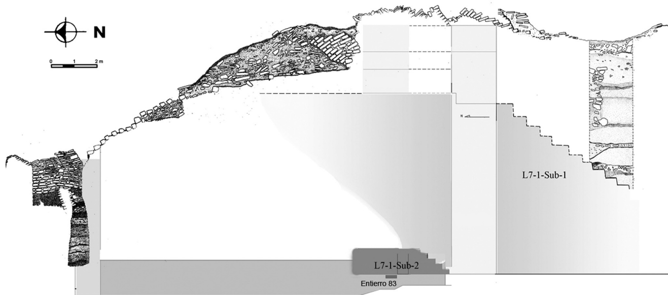
Fig.6: Perfil oeste del palacio de Cancun, en su eje central, mostrando las subestructuras L7-1-Sub-2 y L7-1-Sub-1 (Realizado por T. Barrientos y L. F. Luin).
