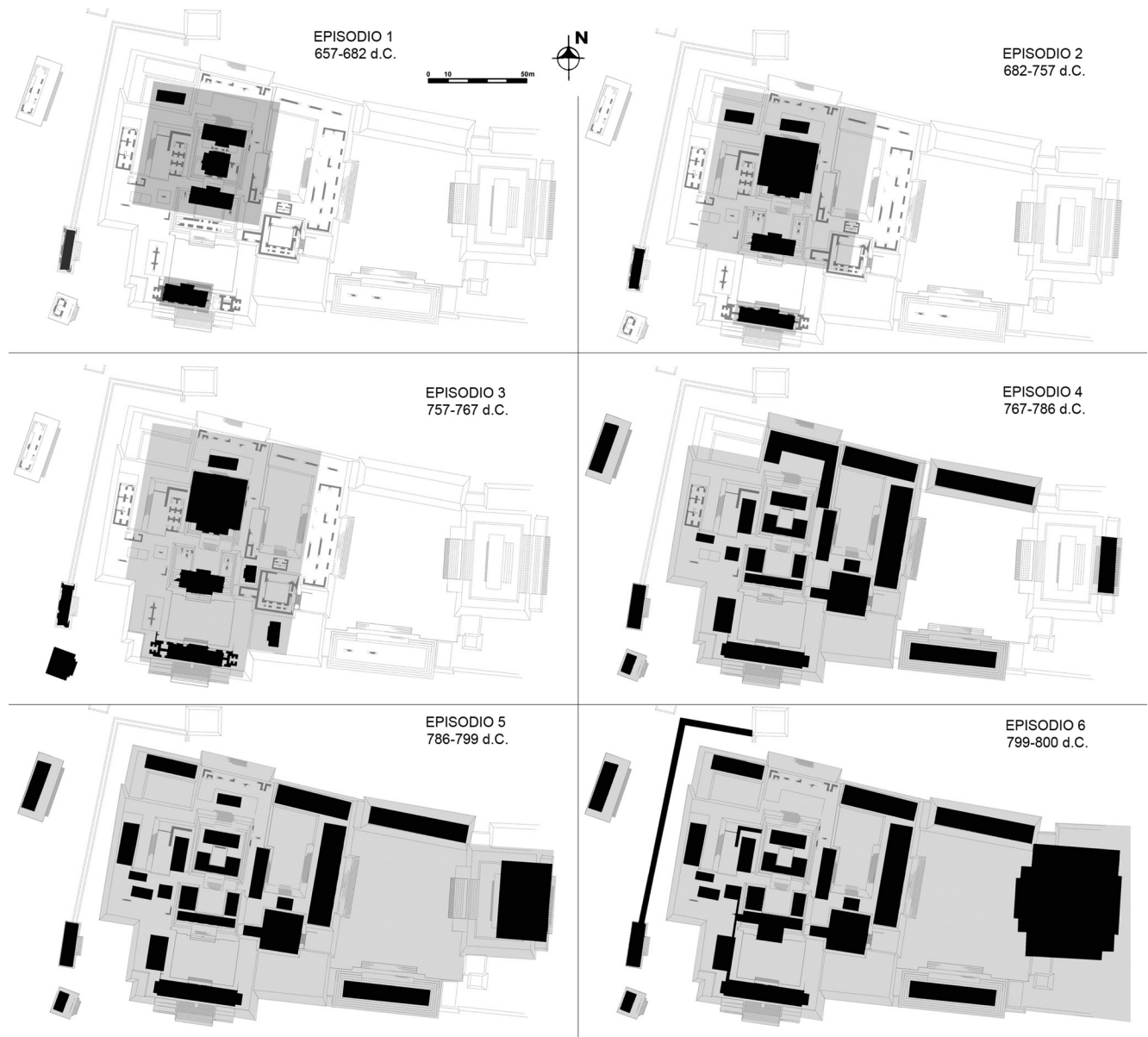
Fig.5: Plano del palacio de Cancun, mostrando la ubicación de estructuras correspondientes a sus seis episodios constructivos (Realizado por T. Barrientos y L. F. Luin).
