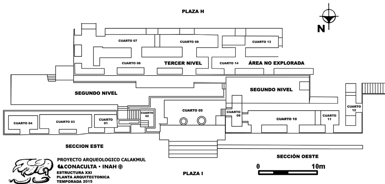
Figura 5. Planta arquitectónica de la Estructura XXI ubicando sus diferentes niveles y cuartos, año 2015. Dibujado de María del Sol Ochoa Mendoza y Eduardo Salvador Rodríguez.
