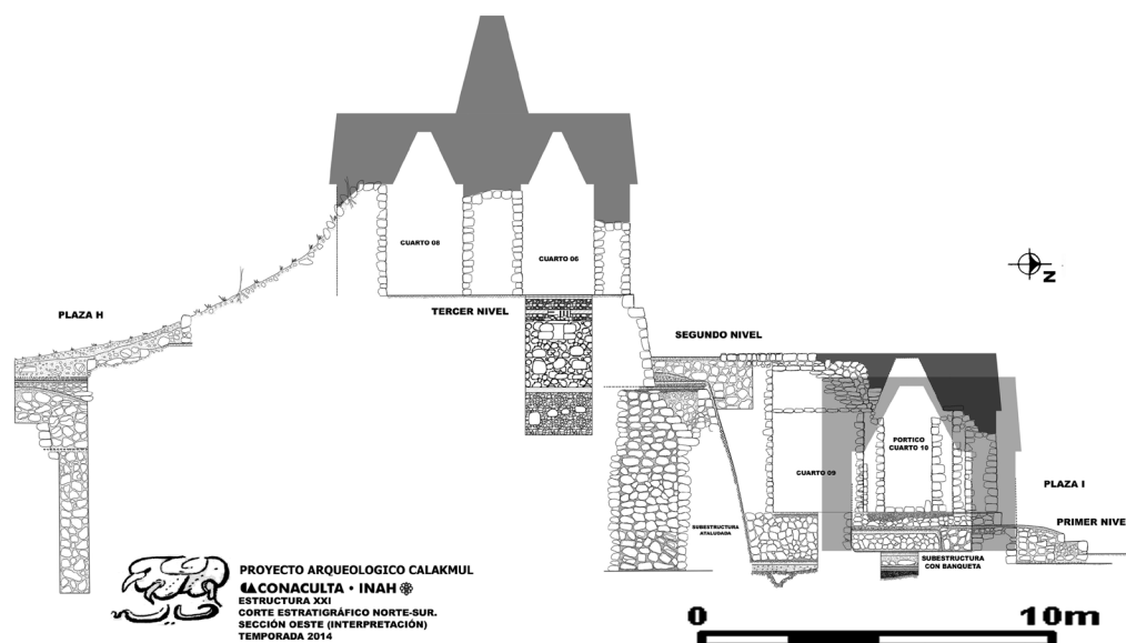
Figura 3. Corte arquitectónico Este-Oeste de la Estructura XXI con interpretación reconstructiva, costado oeste. Dibujo de Eduardo Salvador Rodríguez.
