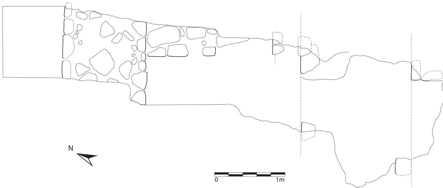
Figura 17b WK06D-56 Planta de Unidad Dibujo de Laura Gámez y David Lee
