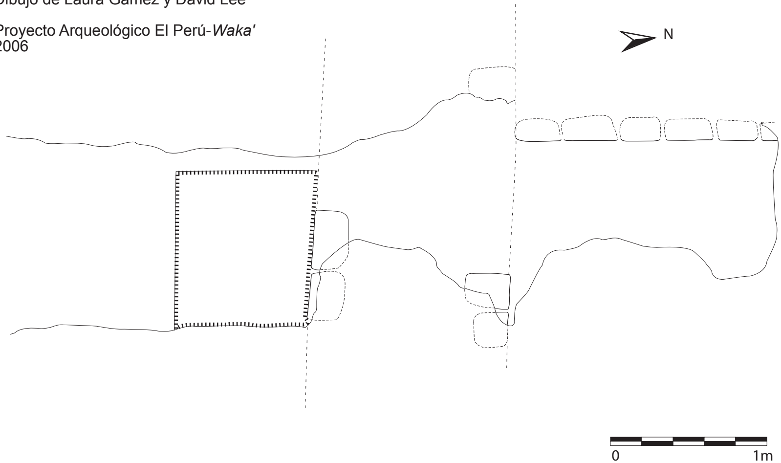
Figura 20b WK06D-60 Planta Dibujo de Laura Gámez y David Lee
